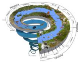
diagrama que muestra las eras geológicas de la Tierra
